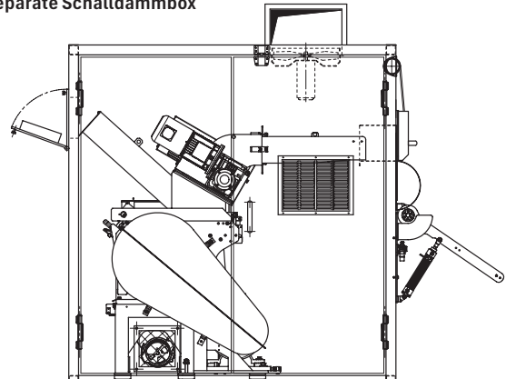
separate Schalldämmbox
