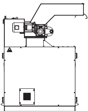
angebaute Schalldämmung
