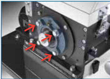
Lagerung direkt an der Mahlkommer befestigt
